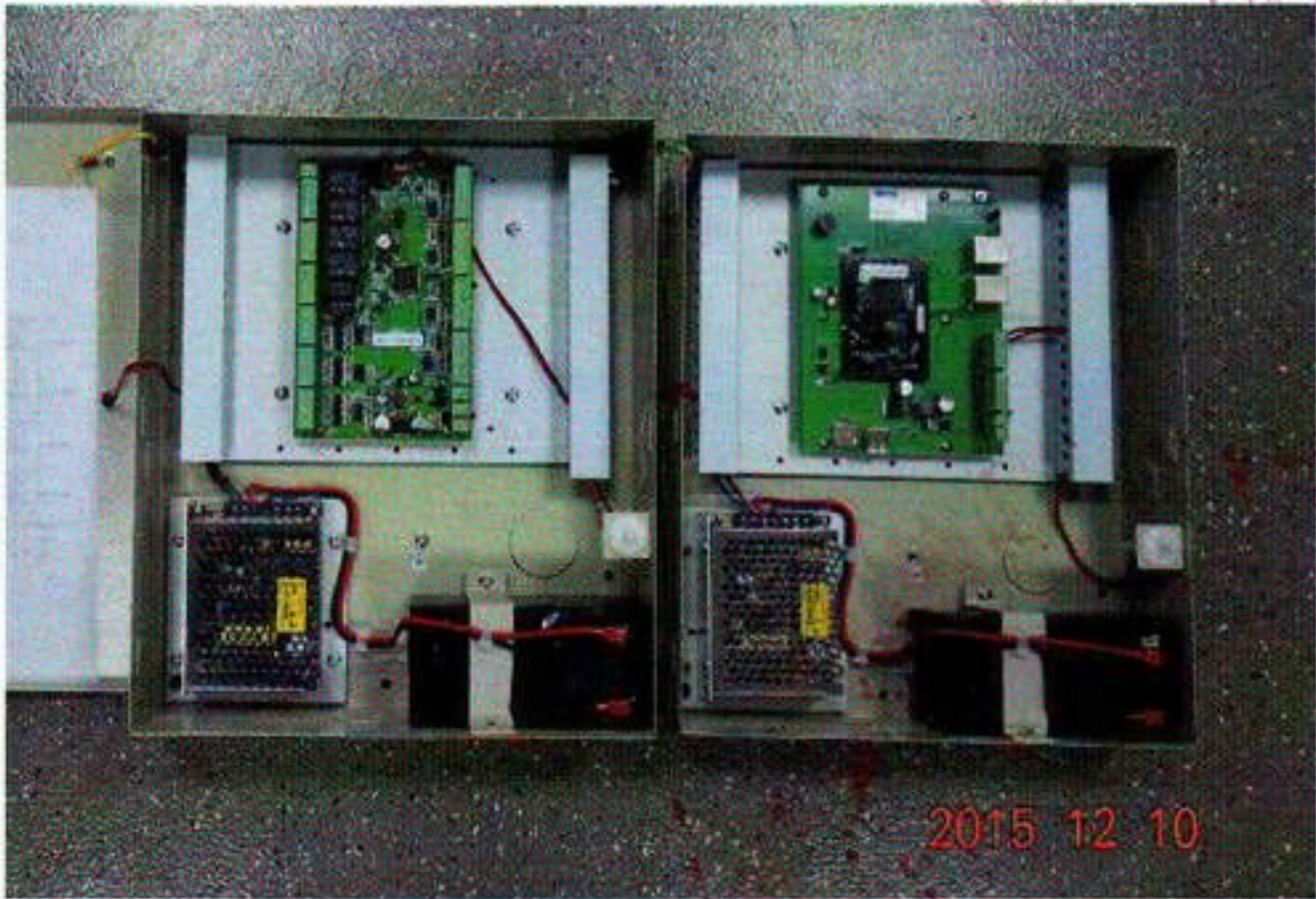
图二、NAC-NCTR 型 网络型门禁控制器样品内部结构
